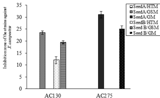
شکل ۱. فعالیت ضد میکروبی سویه‌های استرپتومایسس AC130 و AC275 در برابر X. campestris در محیط پیش‌کشت و تخمیری بر حسب میلی‌متر. محیط پیش‌کشت A و B: (Seed A/B)، محیط‌های تخمیری: هیکی ترزنر (HTM)، گلیسرول سویا (GSM) و گلیسرول (GM).
