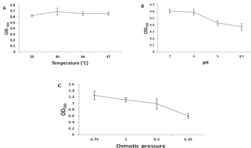
شکل ۱. شرایط بهینه تولید بیوفیلیم در باکتری B. subtilis (A: دما، B: pH و C: فشار اسمزی)
