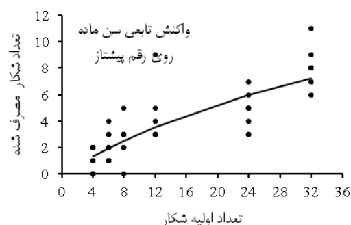
شکل ۲- واکنش تابعی سنک ماده و پوره‌ی سن سوم Orius albipennis در برابر تراکم‌های مختلف شته‌ی جو Sipha maydis روی سه رقم گندم.
